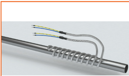
VARMEKABEL HØJTEMP. 450C
